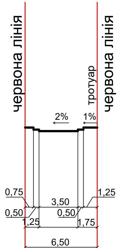
Розріз "Б-Б"
