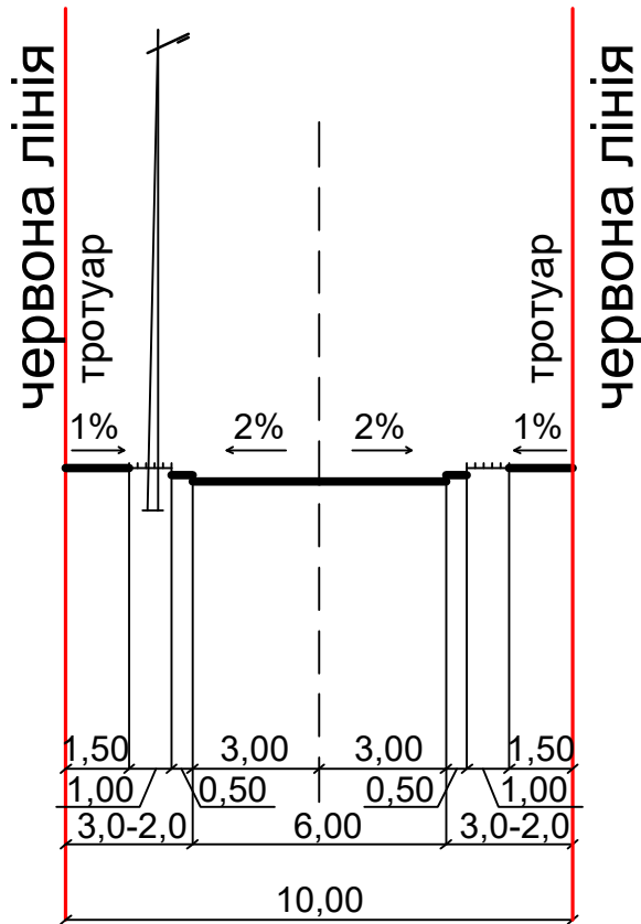
Розріз "А-А"
